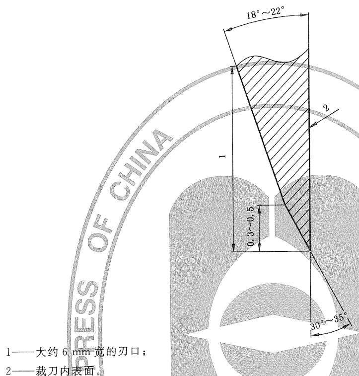
图1 裁刀刃口
